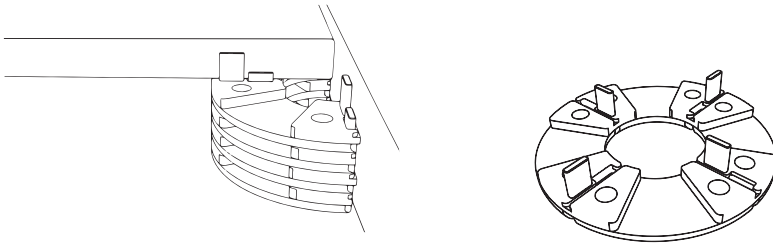
Randlösungen bis 4 cm Aufbauhöhe
